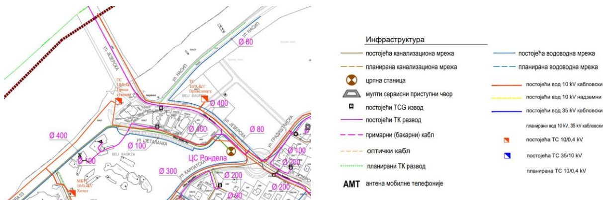
Слика 5. Извод из Измене и допуне Плана детаљне регулације туристичког насеља „Бели Багрем“ општини Велико Градиште, графички прилог бр. 7, Синхрон план инфраструктуре
